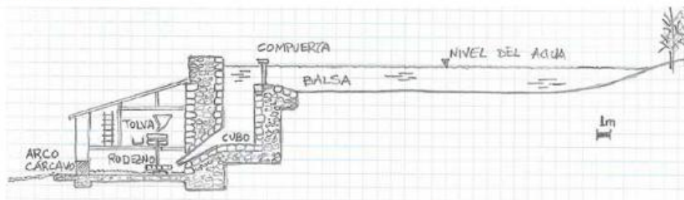
Esquema transversal y elementos principales del Molino Montera
